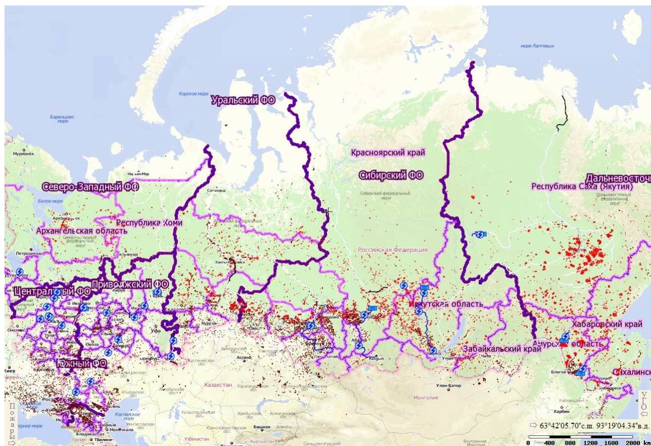
Рис 2.12. Спутниковый мониторинг возникновения термальных точек на территории Российской Федерации в 2011 году
