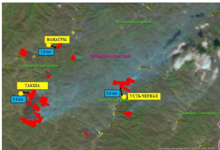
Рис. 2.11. Очаги природных пожаров на территории Забайкальского края
